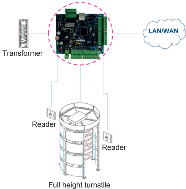
CTRL-1DRTURNSTILE-CF/IP(2.0A)-PCB
