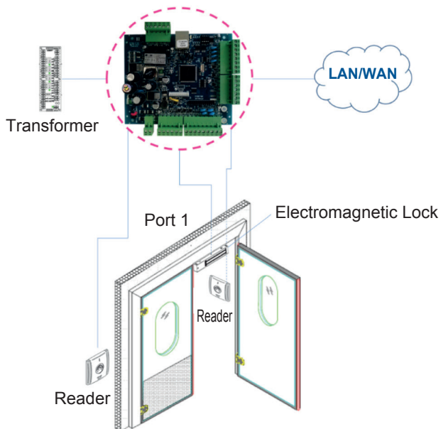
CTRL-1DR-CF/IP(2.0A)-PCB
